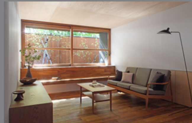
5. HS/8枚建込窓窓 樹種：米松ビラー サイズ：FW3378×FH1998 塗装：Livos タヤシリーズ/チェストナット
