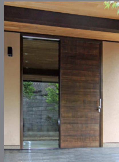
6. E型 1本引・ガラスあり(扉外動) 樹種：タモ 浮作り風仕上げ サイズ：FW1980×FH2782 塗装：Livos カルデットシリーズ/エボニー+クリアー
